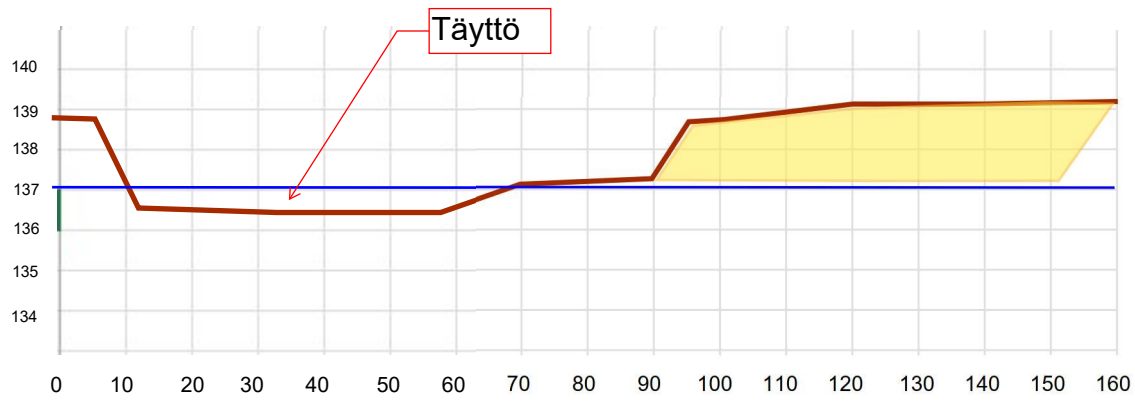
Ylempi ottoalue Leikkaus C-D
